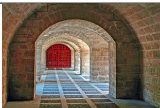
Gewölbe
